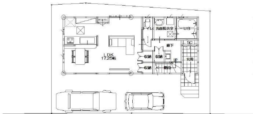
1階 平面図 S:1/100
